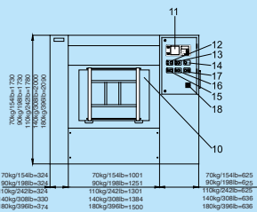
ACHTERKANT MB 70 90 110 140 180
