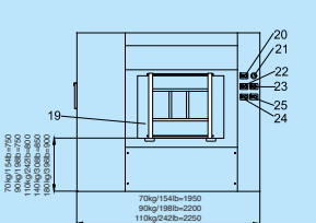
ACHTERKANT MB 70 90 110 140 180
