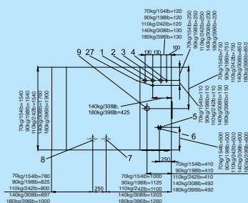
ZIJKANT MB 70 90 110 140 180
